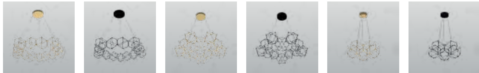
90169/15 медь 1060 × 1060 × 800...1500 мм 69 Вт 3890 лм, 3000 К 90169/15 черный жемчуг 1060 × 1060 × 800...1500 мм 69 Вт 3890 лм, 4000 К 90169/12 медь 850 × 930 × 700...1500 мм 55 Вт 3114 лм, 3000 К 90169/12 черный жемчуг 850 × 930 × 700...1500 мм 55 Вт 3114 лм, 4000 К 90169/5 медь 470 × 470 × 600...1500 мм 25 Вт 1461 лм, 3000 К 90169/5 черный жемчуг 470 × 470 × 600...1500 мм 25 Вт 1461 лм, 4000 К
