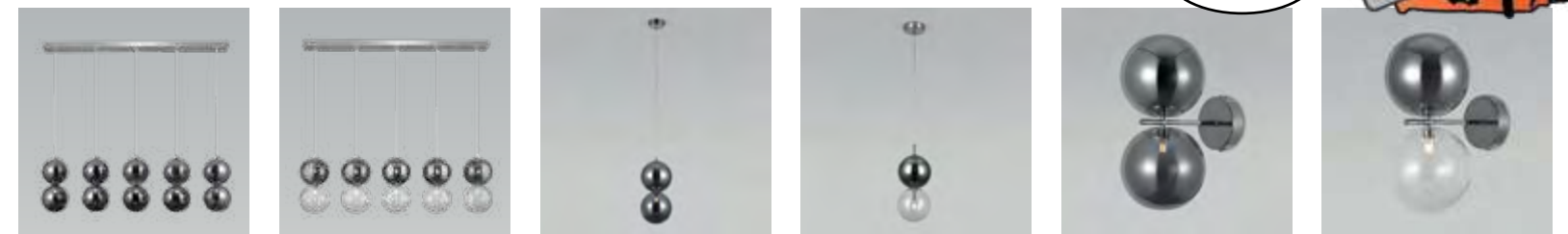
50092/5 хром/дымчатый 1000 × 150 × 380...1500 мм 5 × 3 Вт G4 50091/5 хром/дымчатый 1000 × 150 × 400...1500 мм 5 × 3 Вт G4 50092/1 хром/дымчатый 150 × 150 × 380...1500 мм 1 × 3 Вт G4 50091/1 хром/дымчатый 150 × 150 × 380...1500 мм 1 × 3 Вт G4 50292 хром/дымчатый 150 × 220 × 330 мм 1 × 3 Вт G4 50291 хром/дымчатый 150 × 220 × 330 мм 1 × 3 Вт G4
