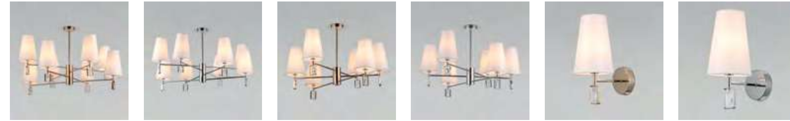
60137/8 золото 900 × 900 × 505 мм 8 × 40 Вт E14 60137/8 хром 900 × 900 × 505 мм 8 × 40 Вт E14 60137/6 золото 700 × 700 × 465 мм 6 × 40 Вт E14 60137/6 хром 700 × 700 × 465 мм 6 × 40 Вт E14 60137/1 золото 210 × 150 × 305 мм 1 × 40 Вт E14 60137/1 хром 210 × 150 × 305 мм 1 × 40 Вт E14
