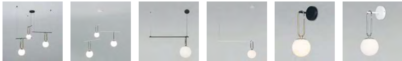
70143/3 черный 970 × 970 × 450...1500 мм 3 × 40 Вт E27 70143/3 белый 970 × 970 × 450...1500 мм 3 × 40 Вт E27 70143/1 черный 950 × 200 × 500...1160 мм 1 × 40 Вт E27 70143/1 белый 950 × 200 × 500...1160 мм 1 × 40 Вт E27 70143 черный 150 × 150 × 425 мм 1 × 40 Вт E27 70143 белый 150 × 150 × 425 мм 1 × 40 Вт E27
